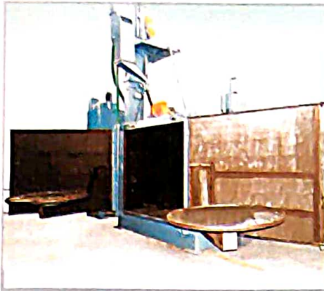
Double Door Type Swing Table Shot Blasting M/c MODEL : AST - 1800
